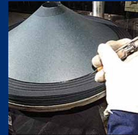
Procedimento di incollaggio bordo/cono.
